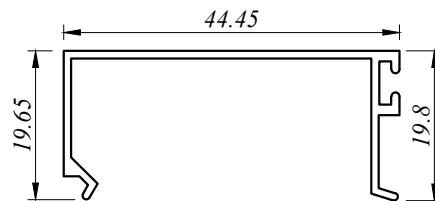
SF 6214 0.268 Kg/M AP : 183.95 MM
