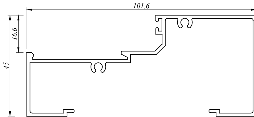
SF 6213 1.045 Kg/M AP : 515.49 MM
