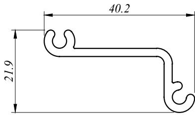
SF 6210 0.380 Kg/M AP : 129.480 MM
