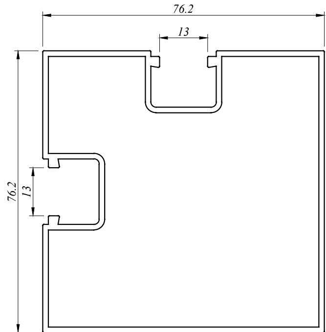
SF 6211 1.565 Kg/M AP : 381.688 MM
