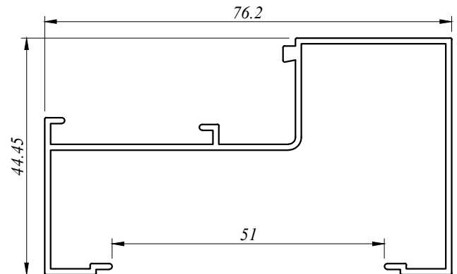
SF 6203 0.653 Kg/M AP : 405.857 MM
