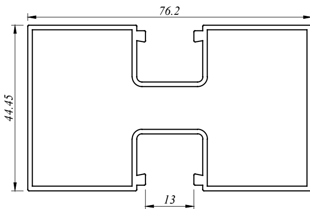
SF 6208 1.076 Kg/M AP : 318.188 MM
