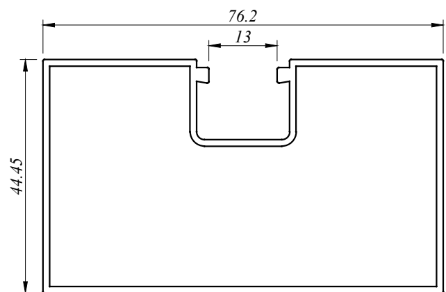
SF 6209 0.965 Kg/M AP : 279.401 MM
