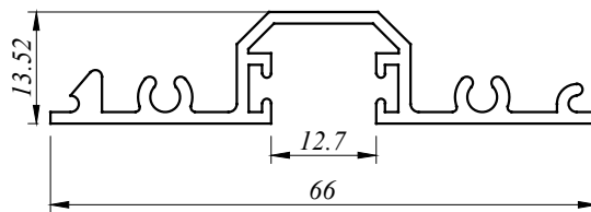
SF 6217 0.534 Kg/M AP : 254.06 MM
