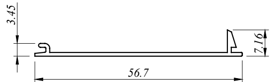
SF 6219 0.195 Kg/M AP : 135.992 MM
