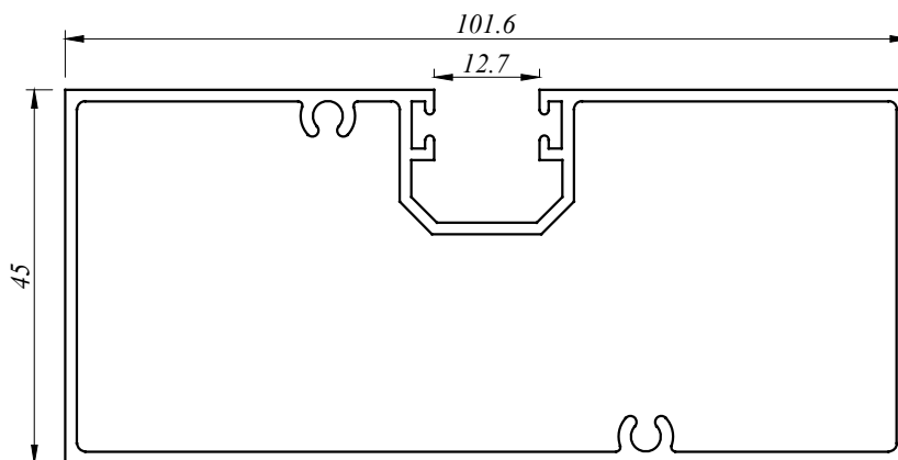
SF 6212 1.378 Kg/M AP : 354.286 MM
