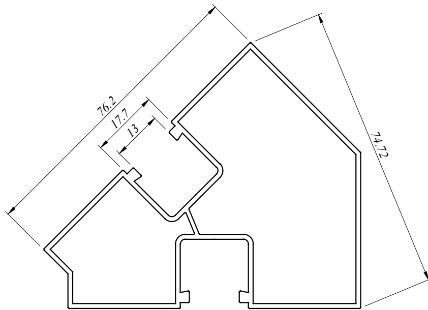
SF 6220 1.193 Kg/M AP : 339.733 MM
