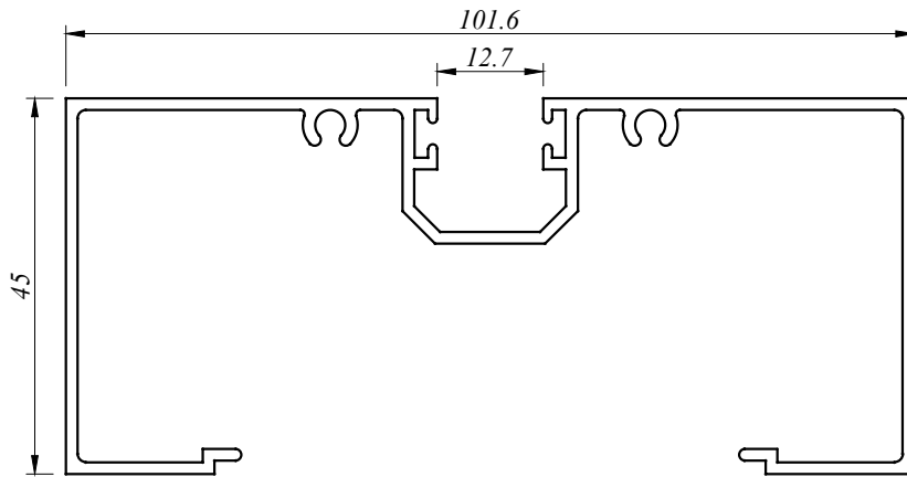
SF 6216 1.156 Kg/M AP : 580.10 MM
