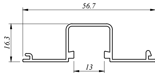
SF 6207 0.340 Kg/M AP : 198.224 MM
