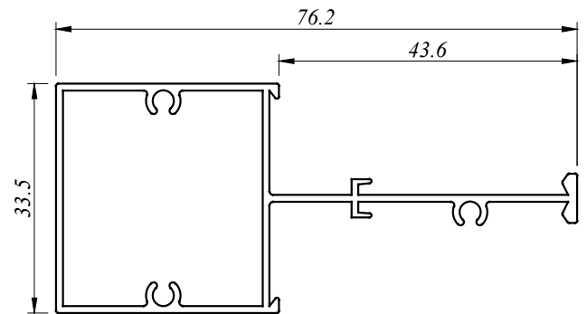
SF 6104 0.599 Kg/M AP : 268.664 MM
