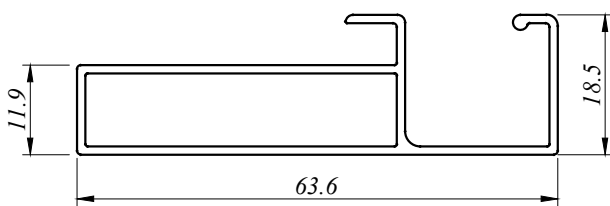
KB 003 0.494 Kg/M AP : 218.969 MM
