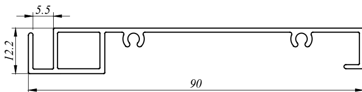
KB 007 0.518 Kg/M AP : 276.716 MM
