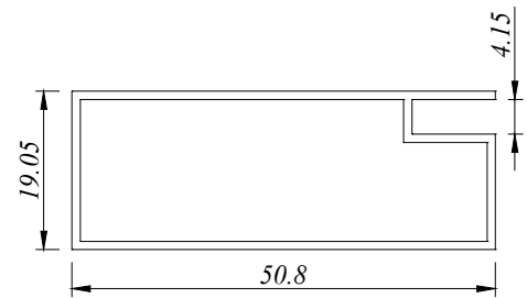
KB 010 0.395 Kg/M AP : 159.700 MM
