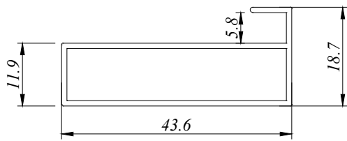
KB 009 0.342 Kg/M AP : 137.456 MM
