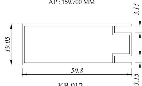
KB 012 0.422 Kg/M AP : 171.70 MM
