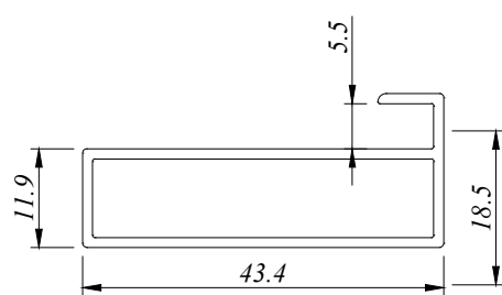
KB 002 H 0.398 Kg/M AP : 135.620 MM
