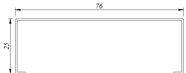
PT 7453 0.288 Kg/M AP : 263.998 MM
