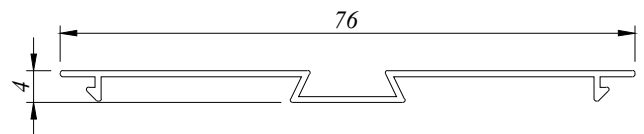
PT 7452 0.210 Kg/M AP : 188.584 MM
