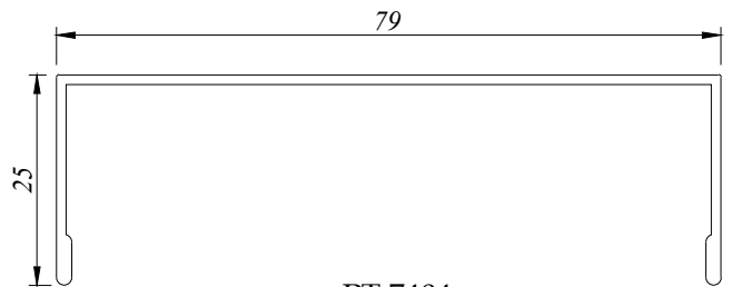
PT 7404 0.427 Kg/M AP : 256.066 MM
