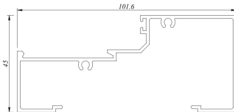
SF 6213 1.045 Kg/M AP : 515.49 MM
