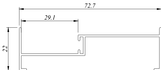
ESD 4203 D 0.382 Kg/M AP : 271.080 MM
