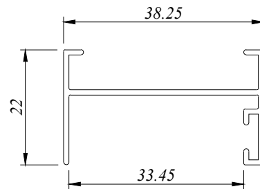
ESD 4210 D 0.289 Kg/M AP : 189.866 MM
