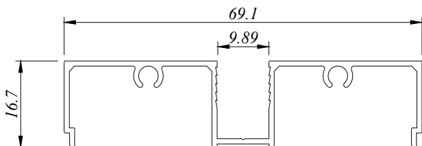
ESD 4212 D 0.451 Kg/M AP : 298.662 MM
