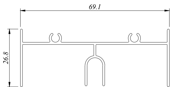
ESD 4201 D 0.496 Kg/M AP : 344.224 MM
