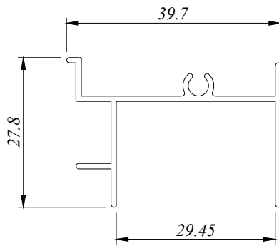
ESD 4209 D 0.325 Kg/M AP : 212.454 MM
