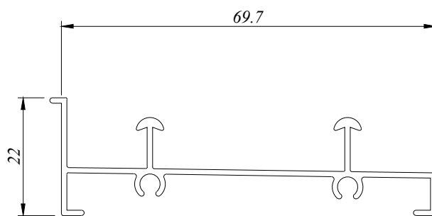
ESD 4202 D 0.450 Kg/M AP : 296.100 MM
