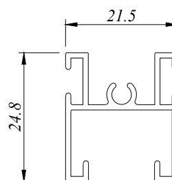
ESD 4204 D 0.300 Kg/M AP : 208.352 MM
