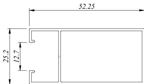
ESD 4205 D 0.457 Kg/M AP : 206.547 MM
