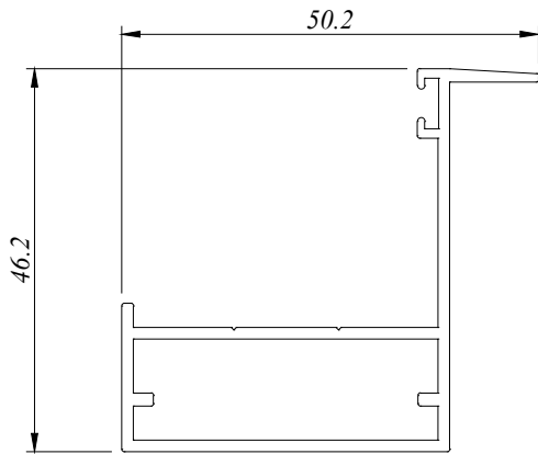
CTW 3716 0.604 Kg/M AP : 196.650 MM
