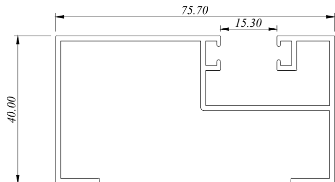
CTW 3707 0.892 Kg/M AP : 465.180 MM
