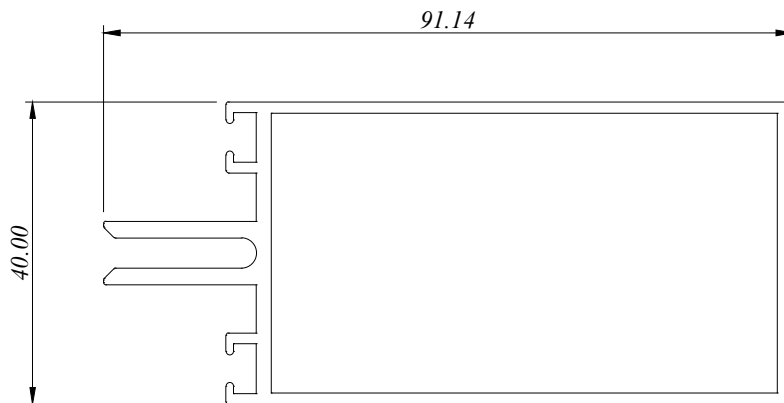
CTW 3710 1.303 Kg/M AP : 340.446 MM
