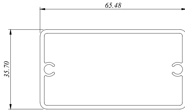
CTW 3713 1.200 Kg/M AP : 197.210 MM
