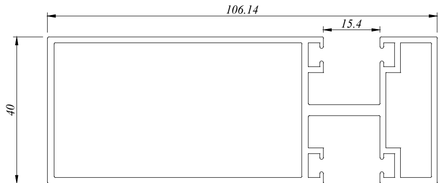
CTW 3709 1.772 Kg/M AP : 435.141 MM
