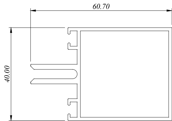
CTW 3702 0.921 Kg/M AP : 279.186 MM
