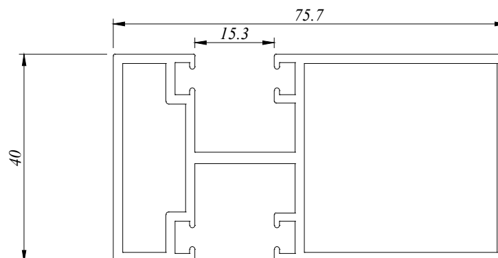
CTW 3711 1.519 Kg/M AP : 370.279 MM
