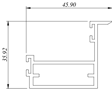
CTW 3708 0.741 Kg/M AP : 196.630 MM
