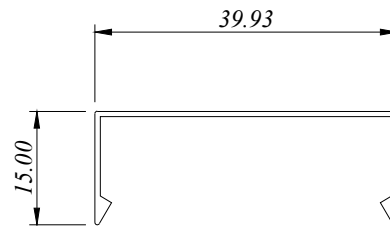
CTW 3704 0.177 Kg/M AP : 140.086 MM
