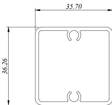
CTW 3705 0.775 Kg/M AP : 138.770 MM
