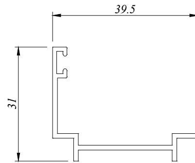
CTW 3717 0.315 Kg/M AP : 184.541 MM
