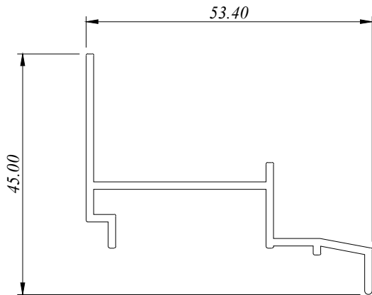
CTW 3701 0.435 Kg/M AP : 233.301 MM
