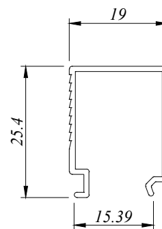
CW 3384 D 0.215 Kg/M AP : 153.376 MM
