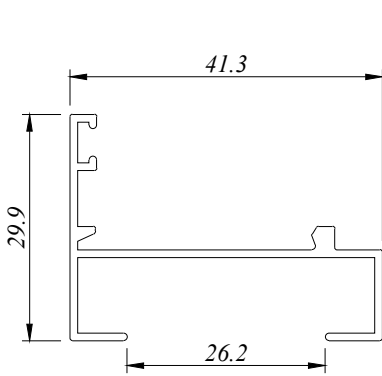
CW 3301 D 0.318 Kg/M AP : 209.062 MM
