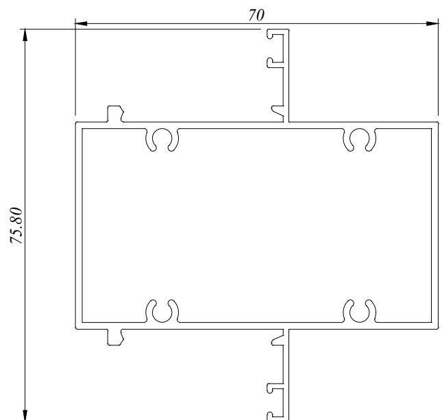
CW 3314 J 1.158 Kg/M AP : 340.049 MM
