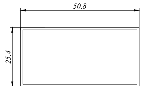
RH 23081610 0.402 Kg/M AP : 151.885 MM
