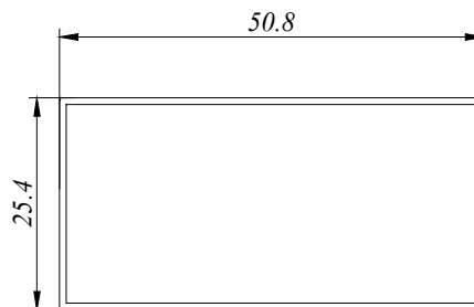
RH 23081608D 0.363 Kg/M AP : 151.885 MM
