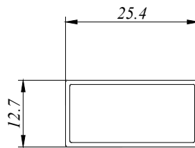
RH 23040814 0.276Kg/M AP : 75.736 MM
