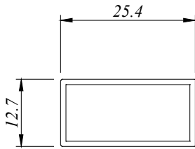
RH 23040810 0.196 Kg/M AP : 75.736 MM
