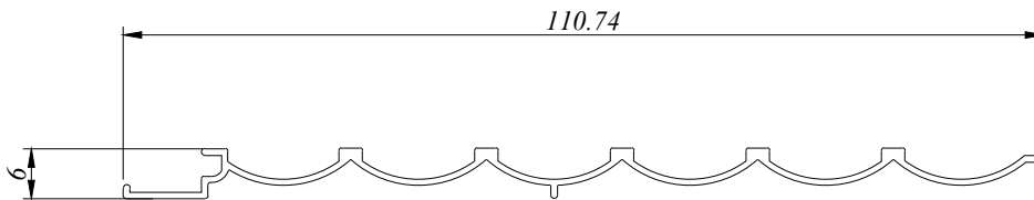
SHC 2208 0.295 Kg/M AP : 266.060 MM
