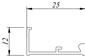
SHC 2205 0.138 Kg/M AP : 90.551 MM
