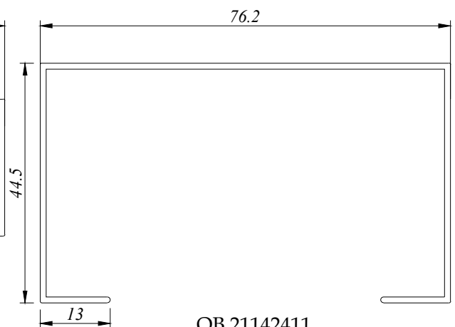
OB 21142411 0.591 Kg/M AP : 375.600 MM
