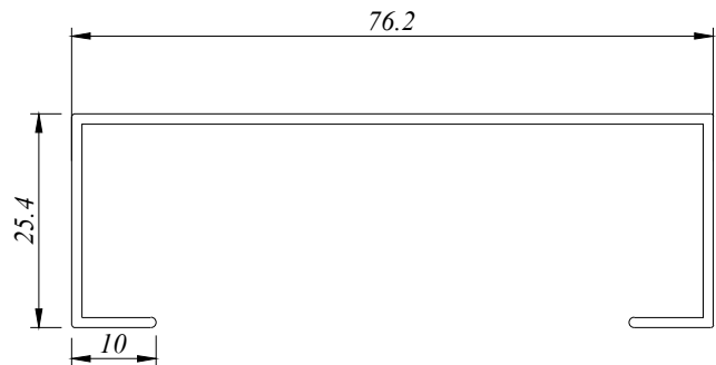
OB 21082412 0.462 Kg/M AP : 288.100 MM
