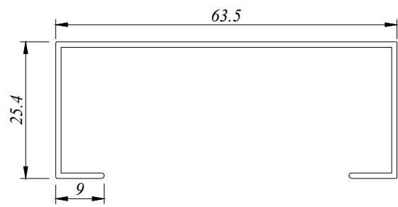
OB 21082010 0.350 Kg/M AP : 262.000 MM
