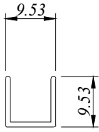
EC 16030309 0.070 Kg/M AP : 54.326 MM
