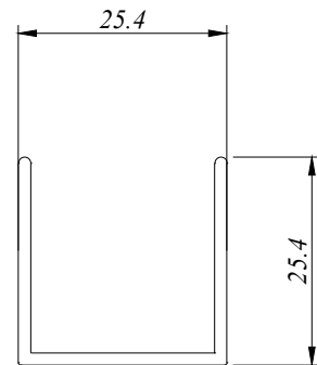
EC 16080815 0.298 Kg/M AP : 148.630 MM
