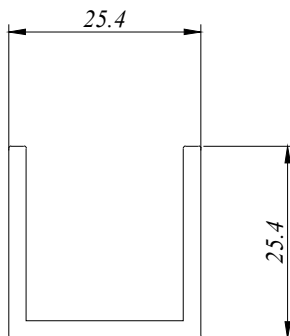
EC 16080825 0.518 Kg/M AP : 147.40 MM
