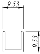
EC 16030310 0.080 Kg/M AP : 54.038 MM
