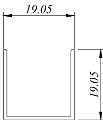
EC 16060609 0.135 Kg/M AP : 111.470 MM
